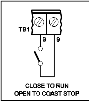
FIG. 7B – ENABLE
